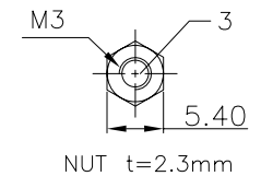
NUT t=2.3mm
