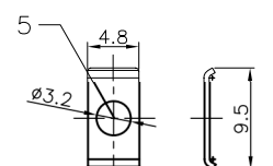
NUT t=2.3mm
